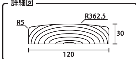
詳細図
